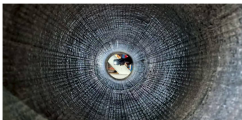
墨西哥项目 纵线工艺耐磨堆焊
